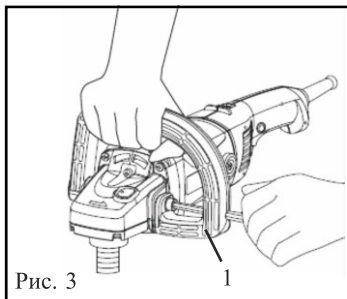
1 – боковая рукоятка
