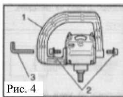
1 - боковая рукоятка; 2 - болт; 3 - ключ шестигранный
